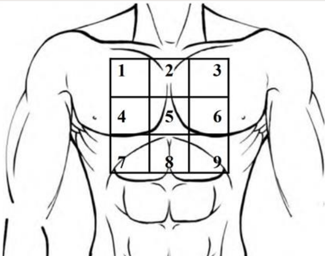
Рис. 7. Процентное распределение ответов на вопрос об алгоритме проведения СЛР – точка компрессии (n=500)
